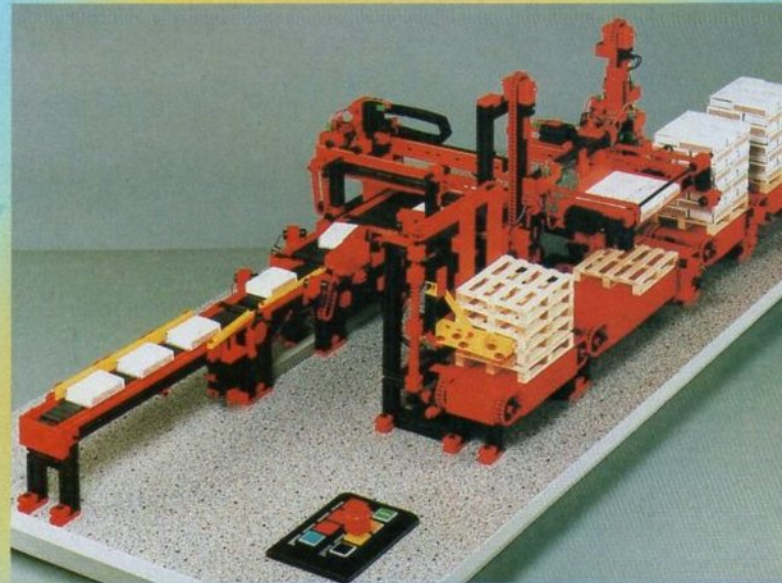
Palettieranlage (Art.-Nr. 35 210)
