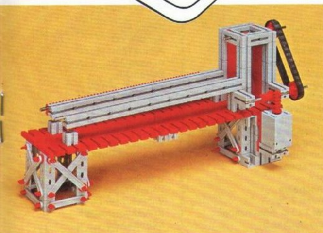
Baustufe 3 In die obere Steinnut werden zur Stabilisierung je 1 Achse 200 und 1 Achse 60 eingeschoben.
