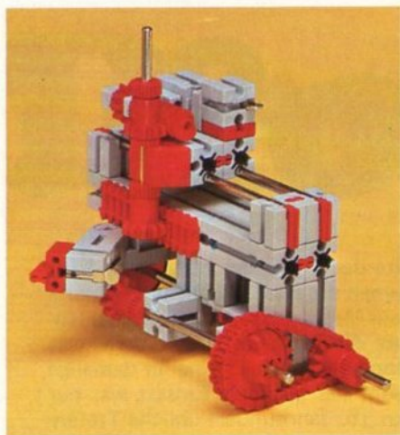
Baustufe 6 Für die Baustufe 6 wurden die Teile der Baustufen 4 und 5 mit Verbindungsstücken 30 zusammengesetzt. Dazu kommt nun der Aufbau des Antriebes, bestehend aus 2 Ritzeln und einer Schnecke. Dieser Antrieb gleitet auf zwei Achsen 110.
