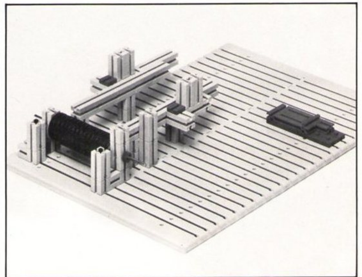
Baustufe 2
