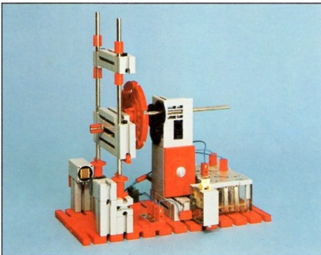
Stanzmaschine mit Lichtschranke. Bauelemente aus u-t1, u-t2, u-t3/1.
