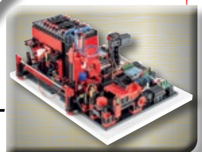
➤ MULTI- BEARBEITUNGS- STATION MIT BRENNOFEN
