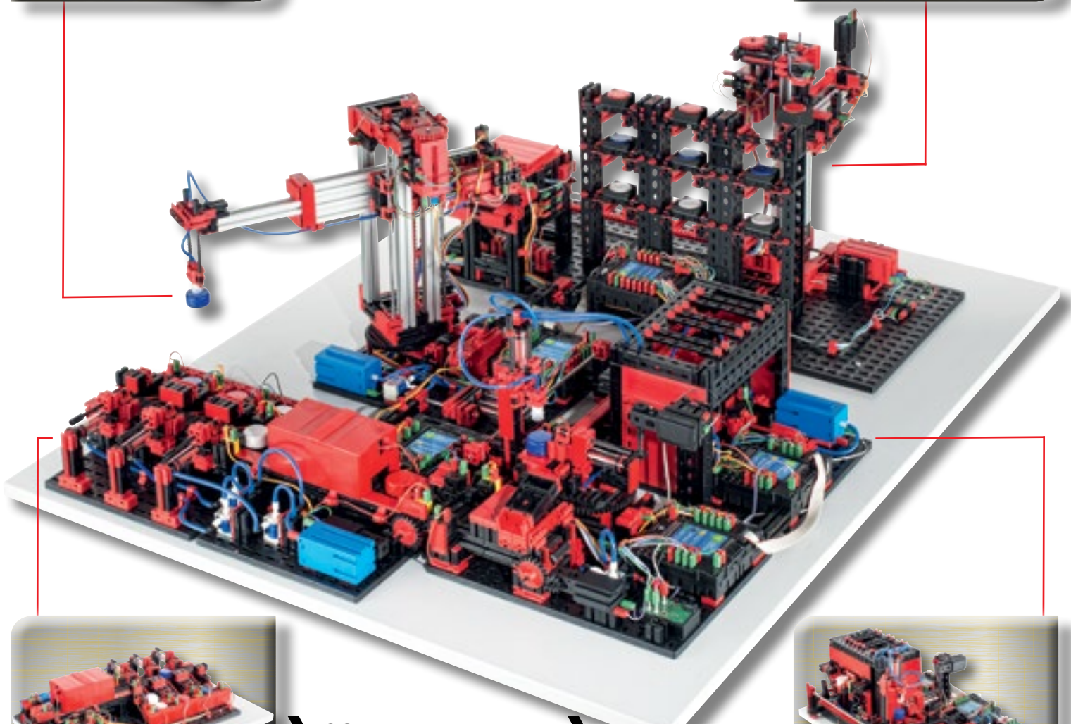
➤ SORTIER- STRECKE MIT FARB- ERKENNUNG
